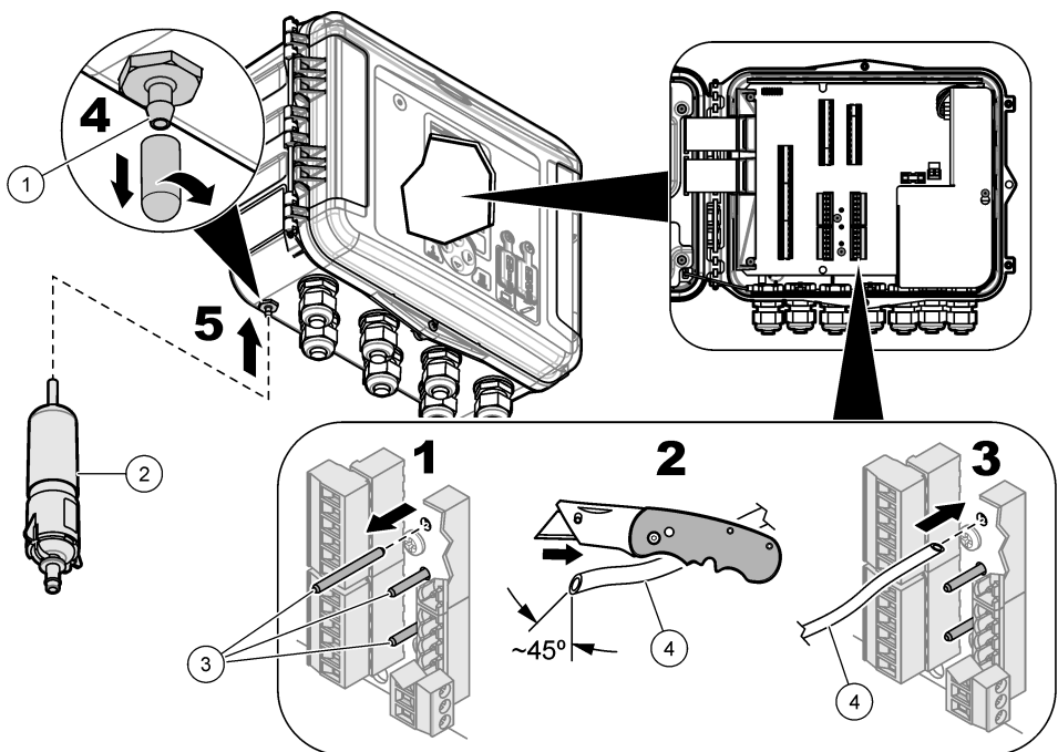
Slika 9 Namestitev referenčne cevke za zrak in sušilnega sredstva
