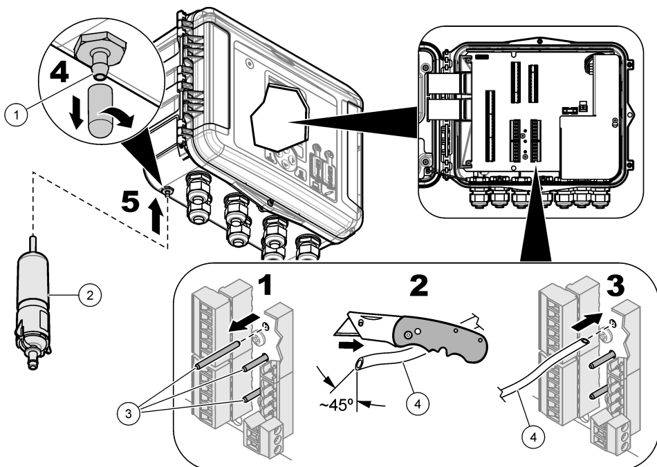
Figur 9 Installation av luftreferensslang och torkmedel
