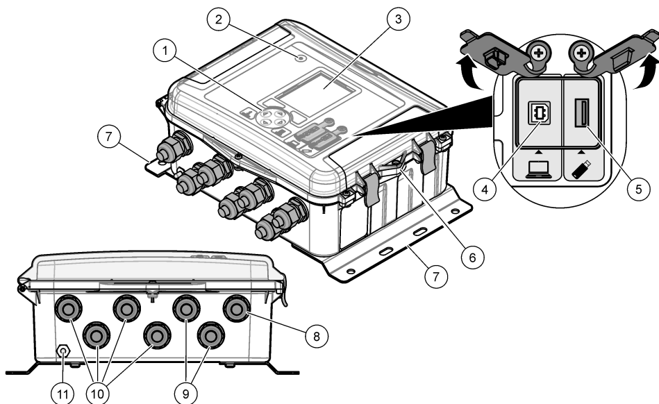
図 1 製品の概要
