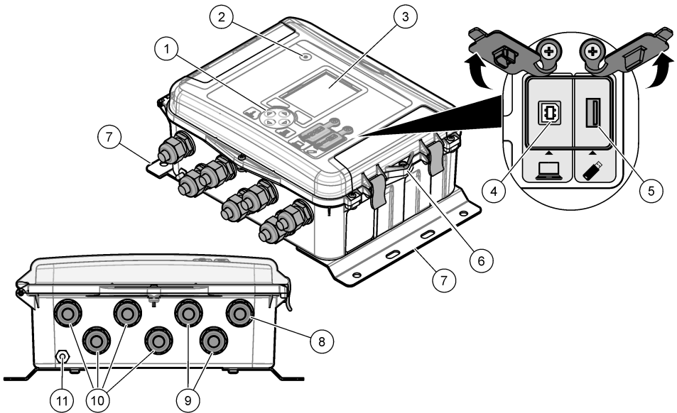
그림 1 제품 개요
