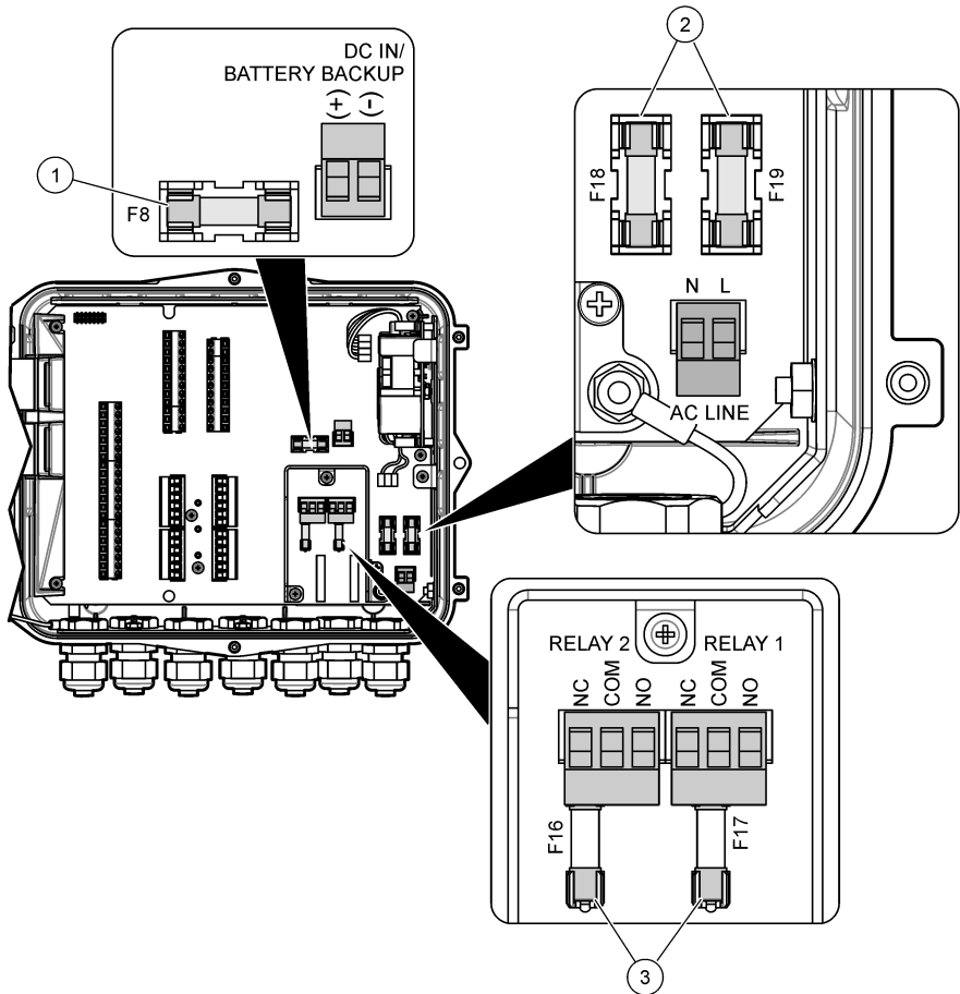
図 12 ヒューズの種類
