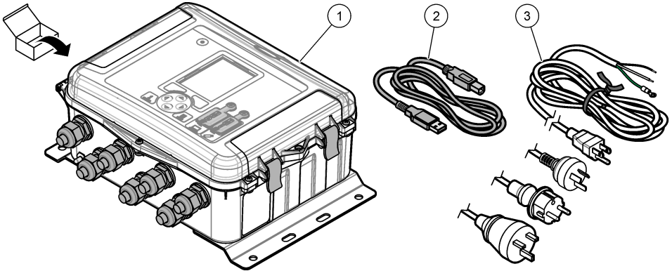
図 2 製品の構成部品
