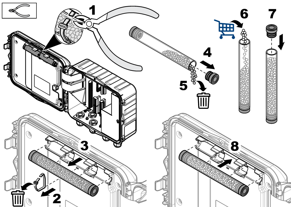
図 13 乾燥剤の交換
