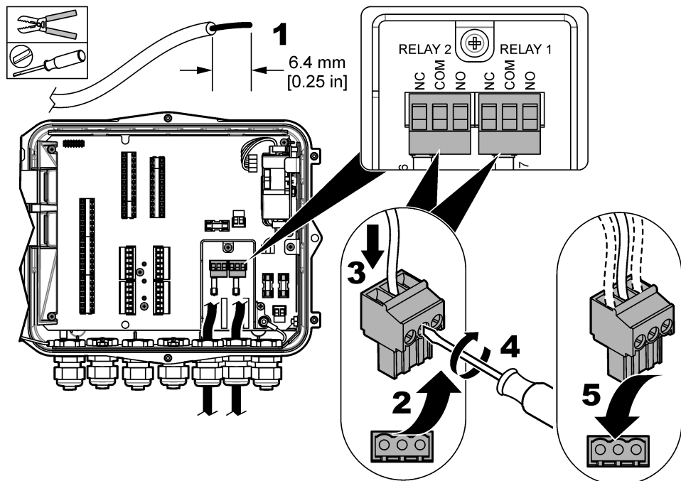
图 10 继电器连接
