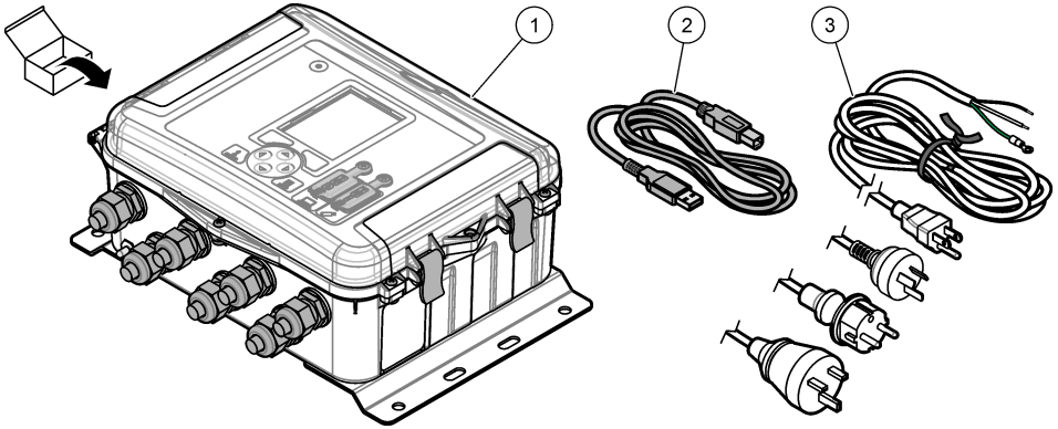
그림 2 제품 구성품
