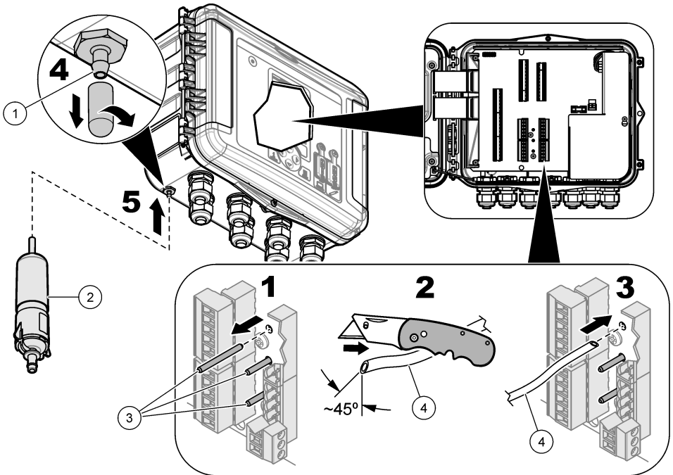
그림 9 공기 참조 튜브 및 건조제 설치
