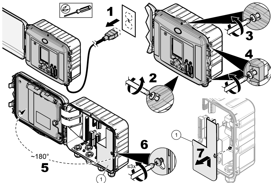
图 5 打开检修门
