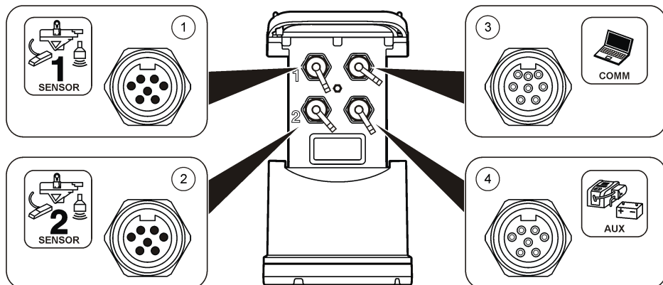
Figure 1 Connecteurs : côté 1
