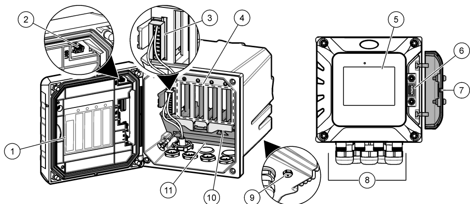
図 1 製品概要
