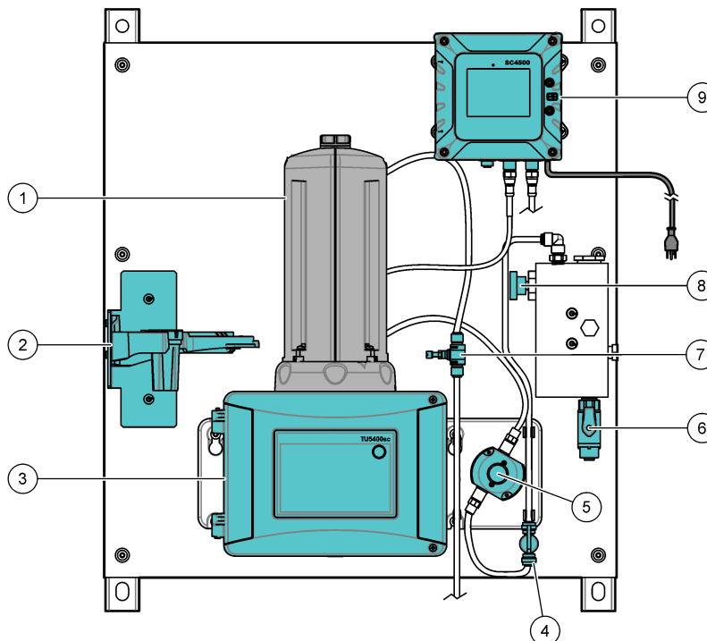
Figure 23 SPMP-TU overview
