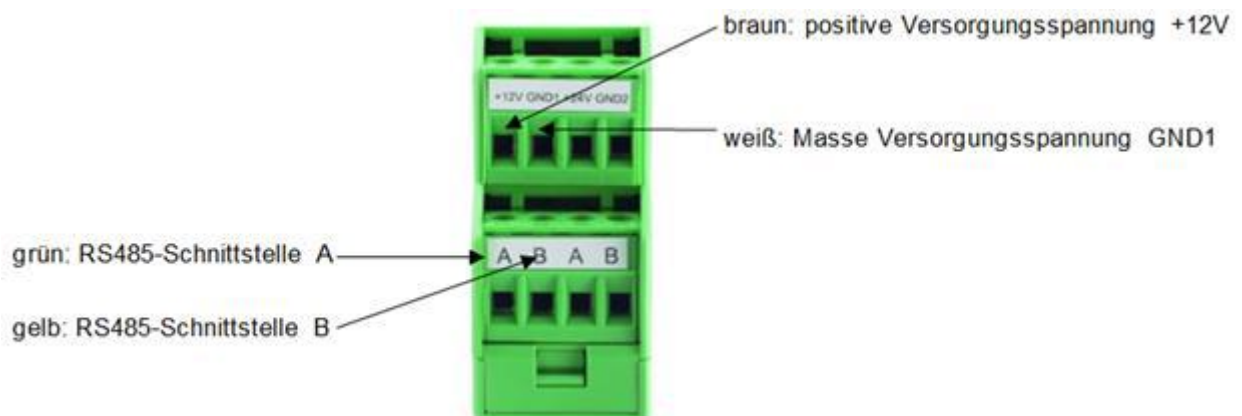
Abbildung 8: Anschluss ISOCON-UMB
