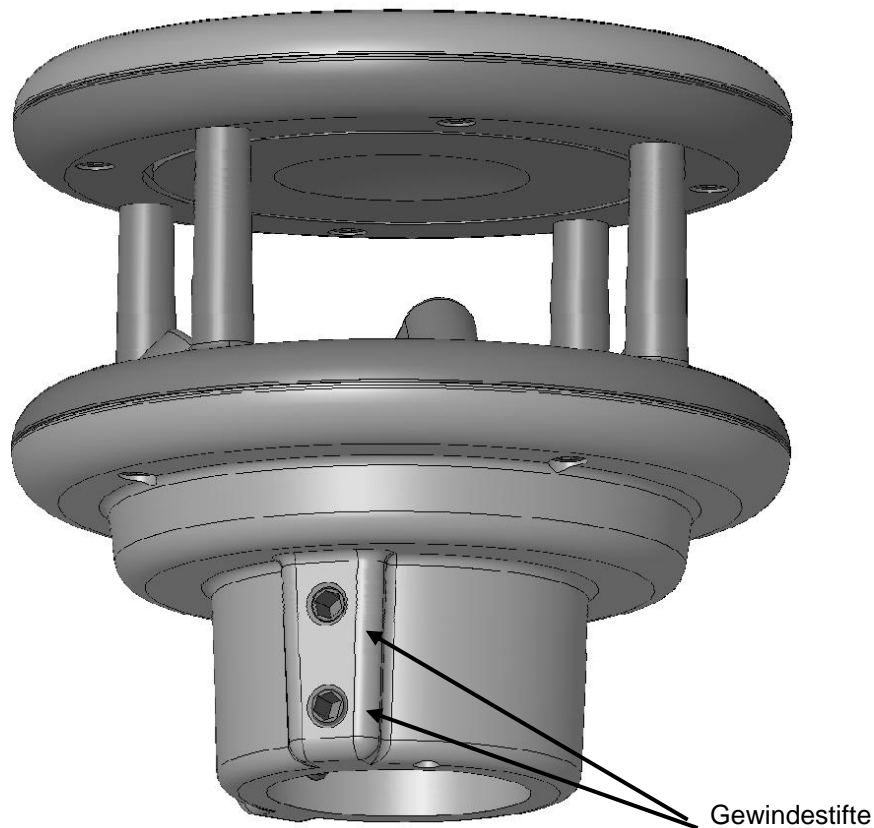
Abbildung 3: Mastbefestigung
