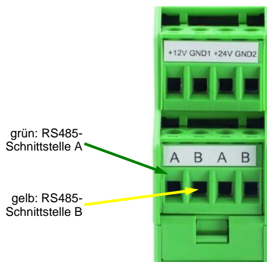
Abbildung 8: Anschluss an Isocon- UMB
