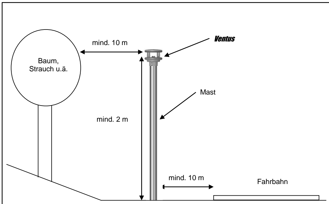
Abbildung 6: Montage-Skizze
